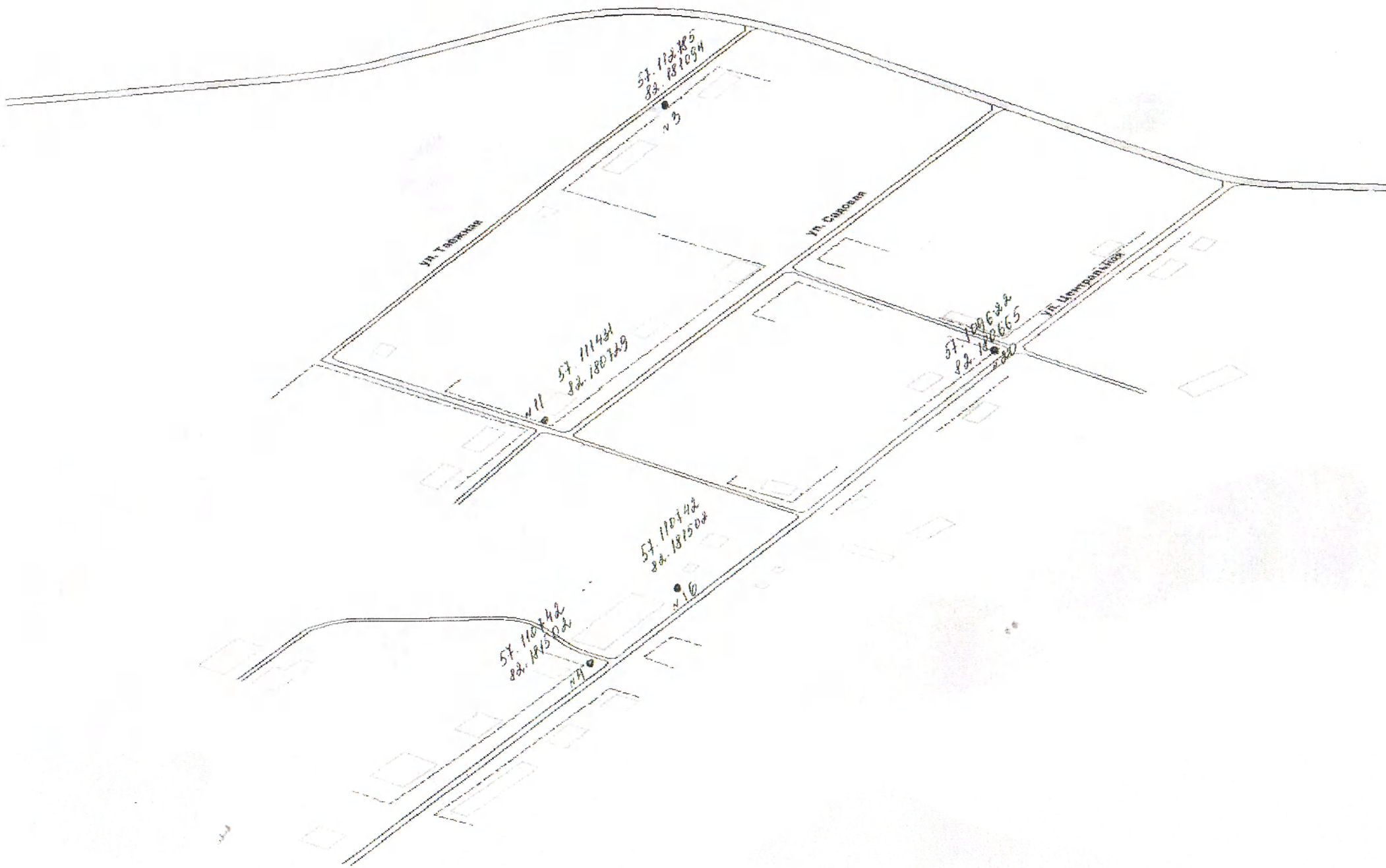
Схема размещения мест (площадок) нахождения твердых коммунальных отходов на территории д. Сухое Бакcharского района Томской области
